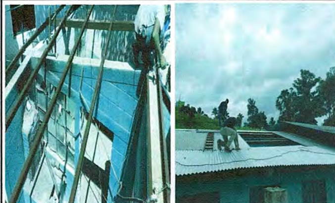
Foto 2: Se inicia con el proceso de cambio de techo en las aulas y la cocina.
